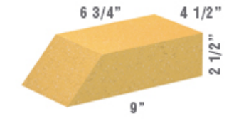
EXTREMO OBLICUO (229-171) x 114 x 63 mm.
