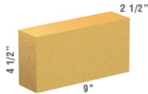
RECTO N°1 de 9" 229 x 114 x 63 mm.
