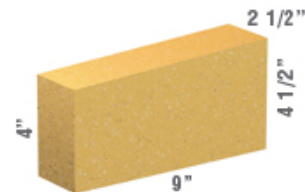
LLAVE N°1 229 x (114-102) x 63 mm.
