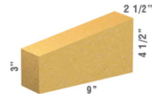
LLAVE N°3 229 x (114-76) x 63 mm.
