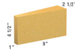
CUÑA N°3 229 x 114 x (63-25) mm.
