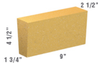
ARCO N°2 229 x 114 x (63-44) mm.
