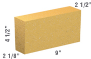
ARCO N°1 229 x 114 x (63-54) mm.
